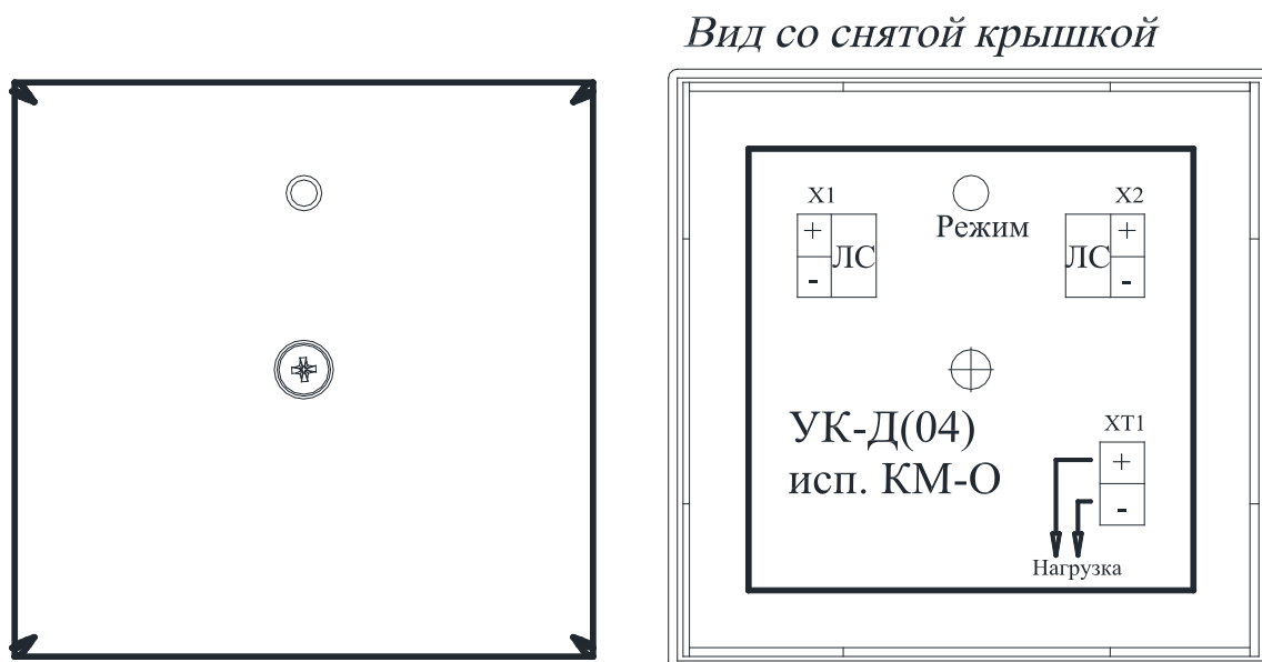
Рис.1 Внешний вид устройства
